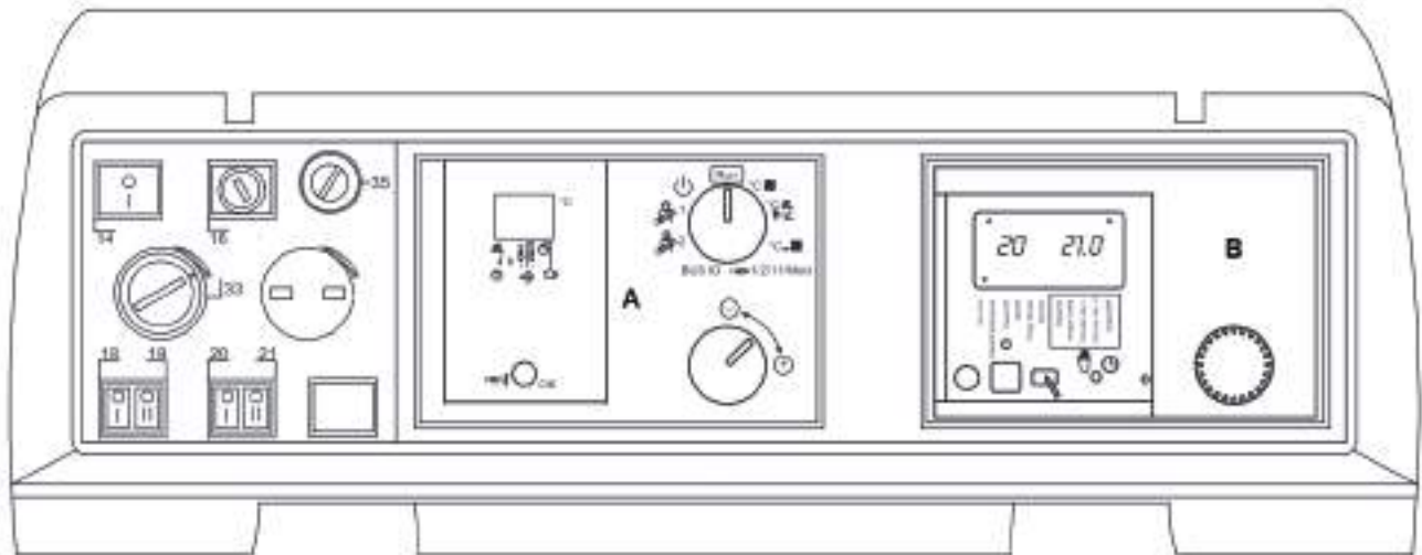
Пульт MASTER (арт. 00373169)
