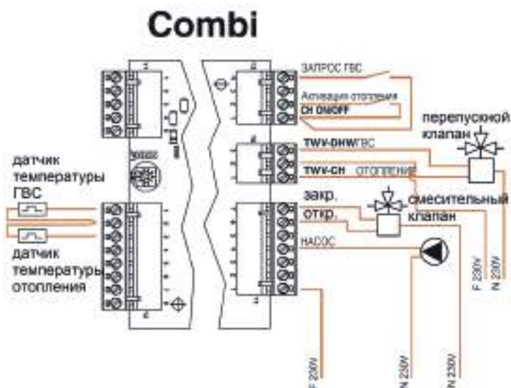
Контур отопления со смесительным клапаном + пластинчатый теплообменник ГВС
