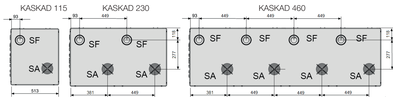
Вид сверху
