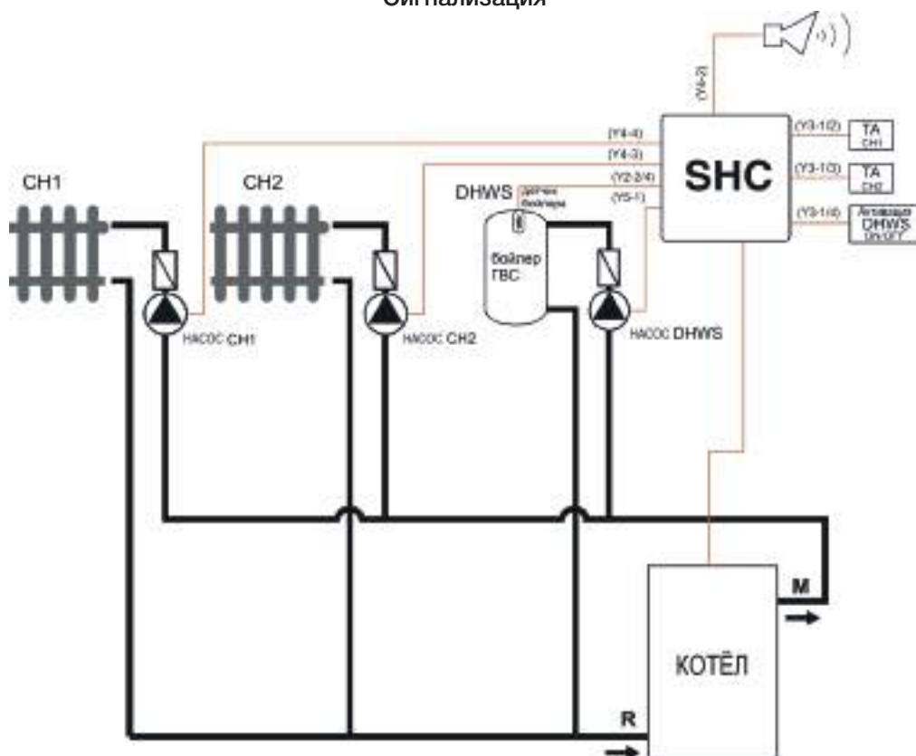
Два прямых контура отопления Бойлер аккумулятор ГВС Сигнализация
