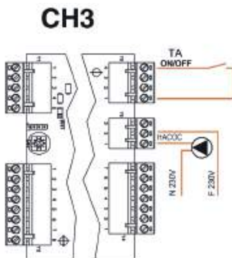
Прямой контур отопления 3
