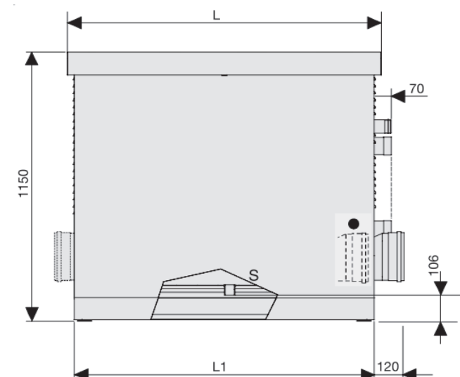
ВИД СБОКУ СЛЕВА
