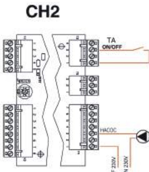
Прямой контур отопления 2
