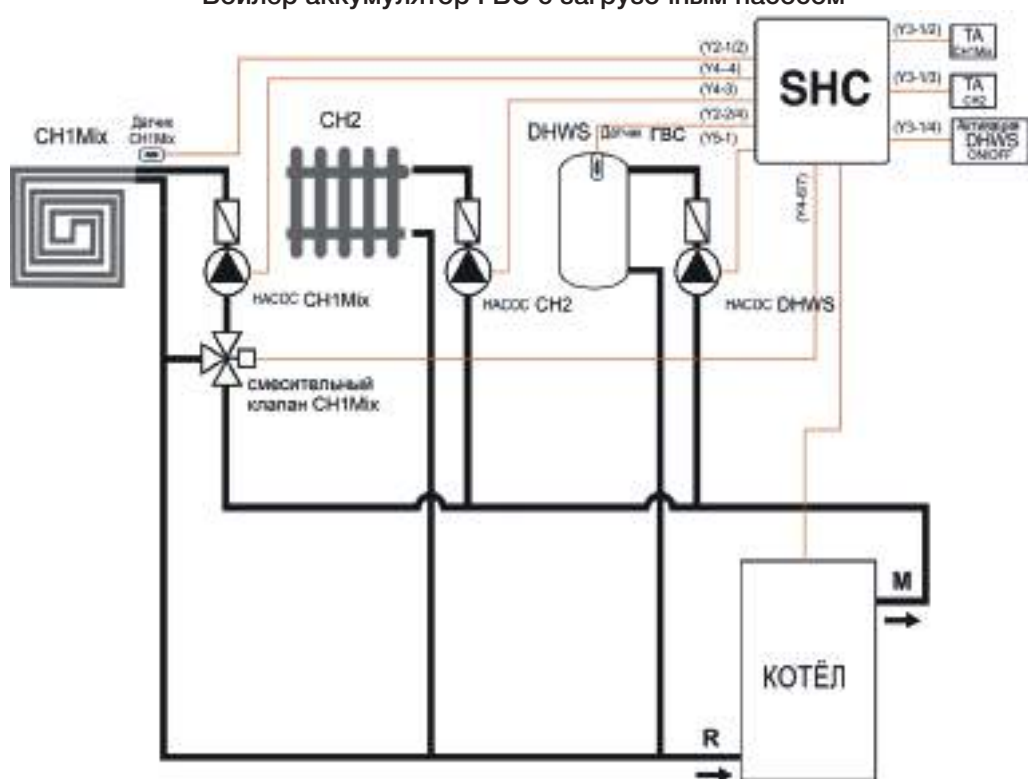
Контур отопления со смесителем Прямой контур отопления Бойлер аккумулятор ГВС с загрузочным насосом
