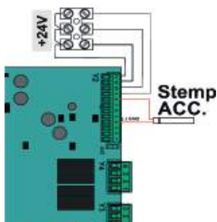
Подключение датчика температуры бойлера ГВС
