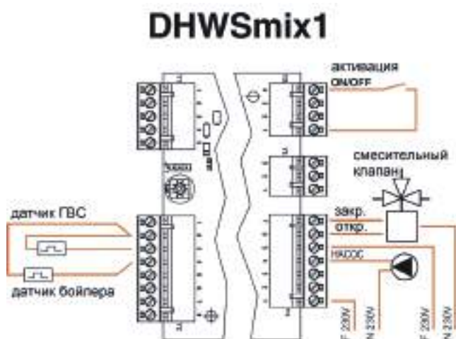
Бойлер ГВС со смесителем на выходе 2
