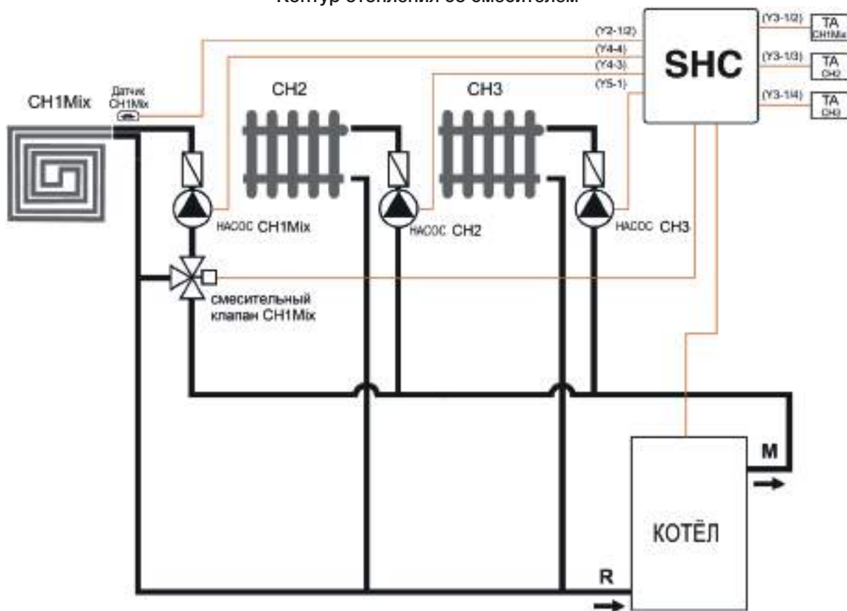
Два прямых контура отопления Контур отопления со смесителем
