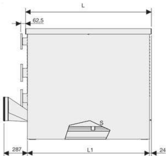
ВИД СБОКУ СЛЕВА
