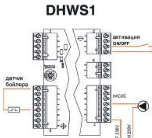
Бойлер ГВС 2
