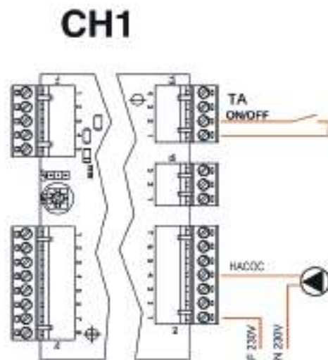
Прямой контур отопления 1
