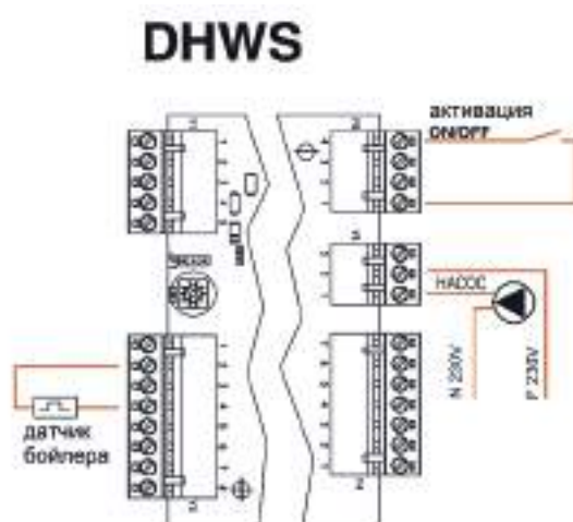
Бойлер ГВС 1
