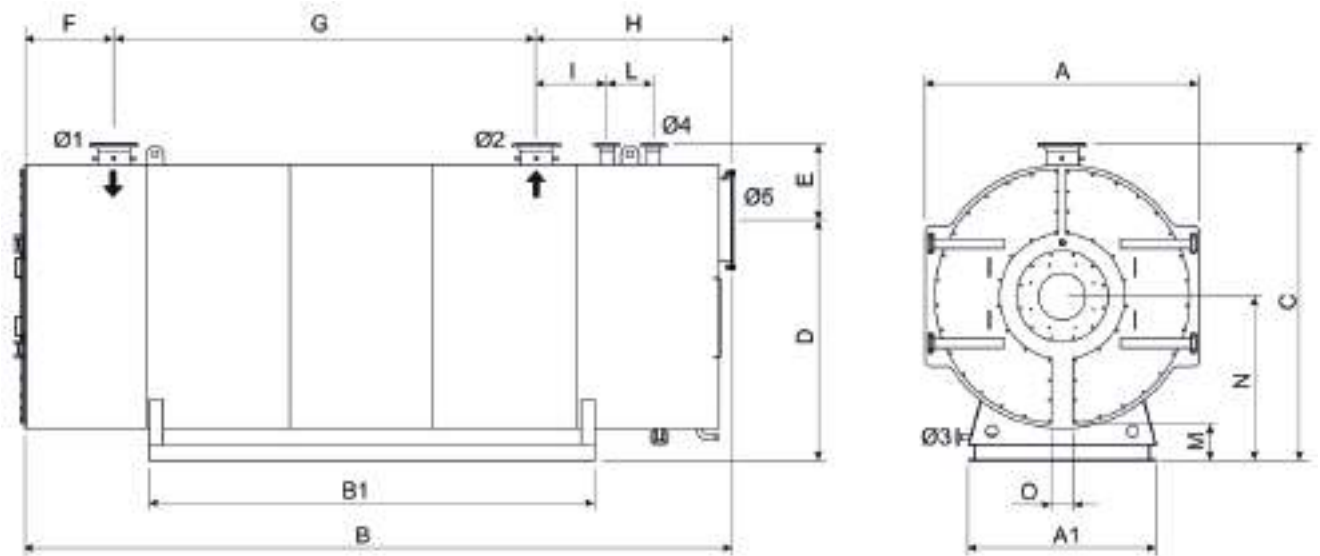
МОДЕЛЬ КОТЛА
