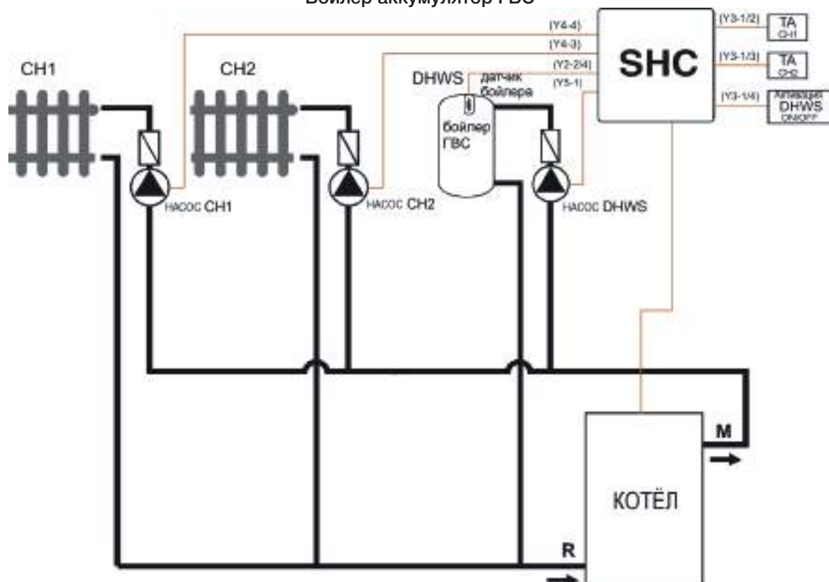
Два прямых контура отопления Бойлер аккумулятор ГВС
