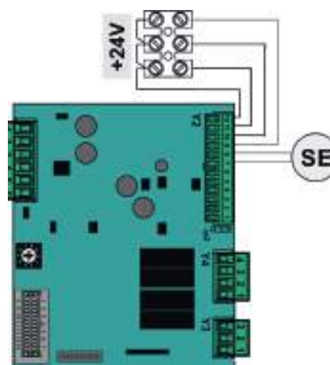
Подключение датчика наружной температуры
