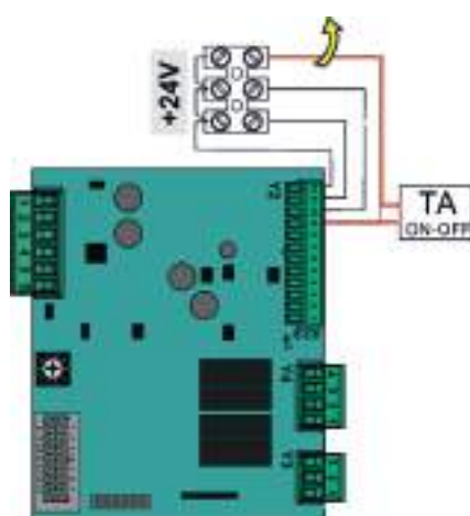
Подключение комнатного термостата
