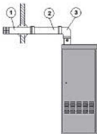
Дымоудаление через боковую стену
