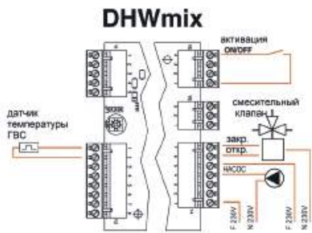
Пластинчатый теплообменник ГВС
