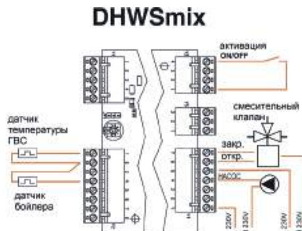
Бойлер ГВС со смесителем на выходе 1
