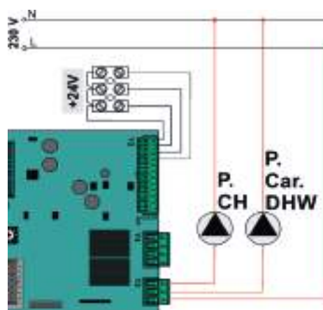
Подключение насоса высокотемпературного контура и загрузочного насоса ГВС
